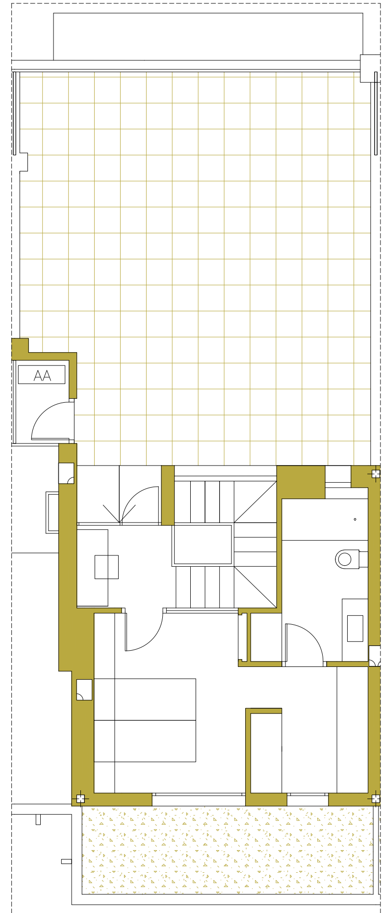
PLANTA TERCERA
